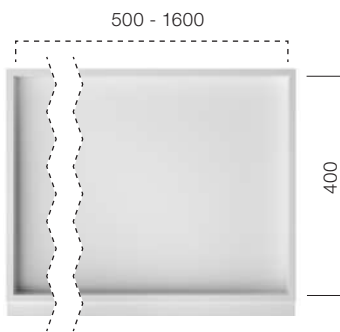
Beckentiefe: 54 mm
