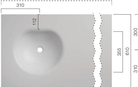
Beckenposition: Links; Beckentiefe: 130 mm
