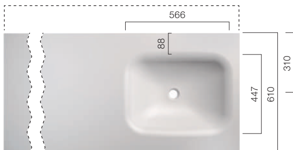
Beckenposition: Rechts; Beckentiefe: 120 mm
