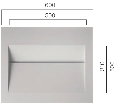
Beckentiefe: 80 mm
