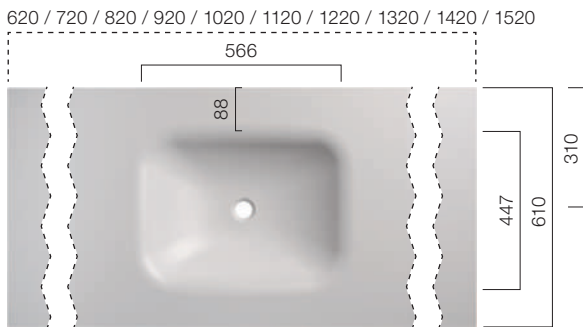
Beckenposition: Mitte; Beckentiefe: 120 mm
