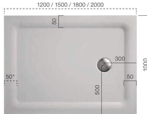
Für den bodengleichen Einbau. *Funktionsrand (individuell kürzbar) ⊗ ⊗ ⊗ ⊗
