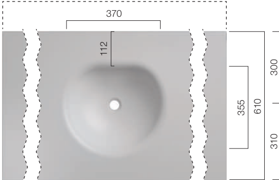
Beckenposition: Mitte; Beckentiefe: 130 mm
