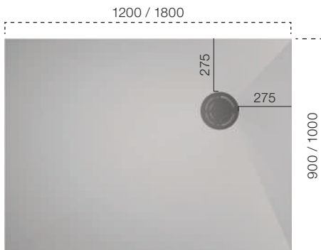
XERO rechteckig – Ablauf dezentral
