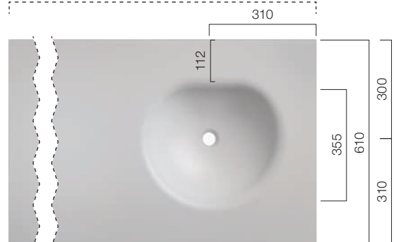
Beckenposition: Rechts; Beckentiefe: 130 mm
