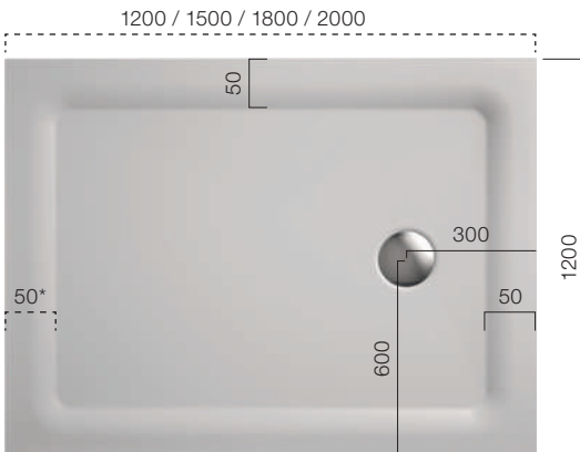
Für den bodengleichen Einbau. *Funktionsrand (individuell kürzbar) ⊗ ⊗ ⊗ ⊗
